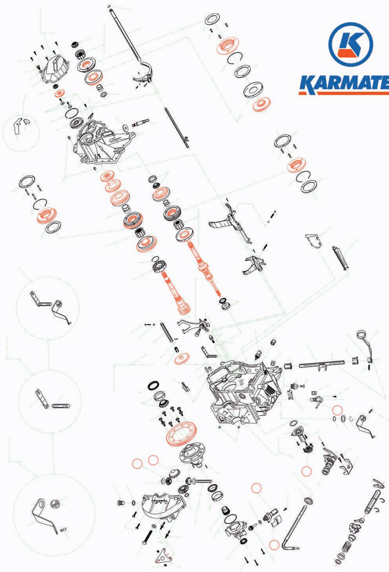
نقشه انفجاری گیربکس پژو PEUGEOT GEARBOX ASSY.
