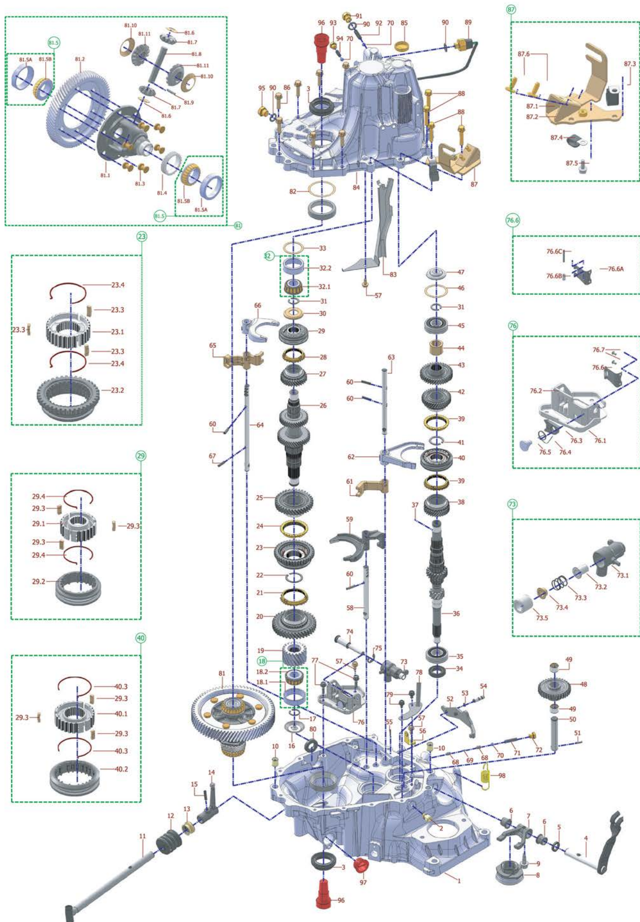
TIBA GEARBOX ASSY. نقشه انفجاری گیربکس تیا
